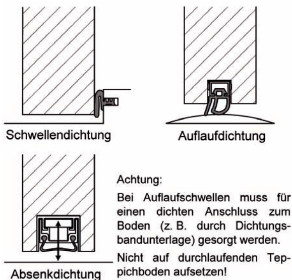
Bild 10 Abdichtungsmöglichkeiten zwischen Tür und Fußboden
