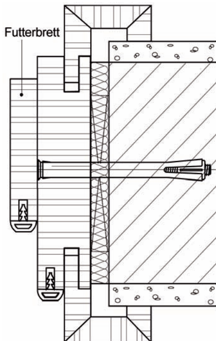
Bild 8 Tüorzarge mit zusätzlicher mechanischer Befestigung
