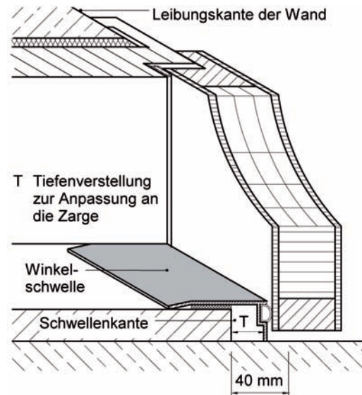
Bild 6 Schwellekante mit ca. 40 mm Rücksperrung gegenüber Leibungskante der Wand
