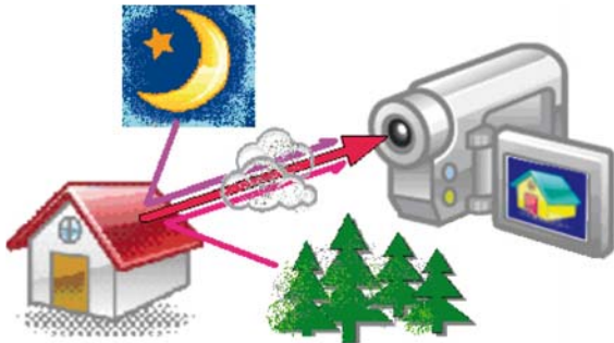
Bild 5 Die von der Thermographiekamera empfangene Strahlung setzt sich aus der emittierten Strahlung und aus Störstrahlung durch Reflexion der Umgebung zusammen. Bei größeren Abständen kann die Strahlung außerdem durch die Atmosphäre verfälscht werden.
