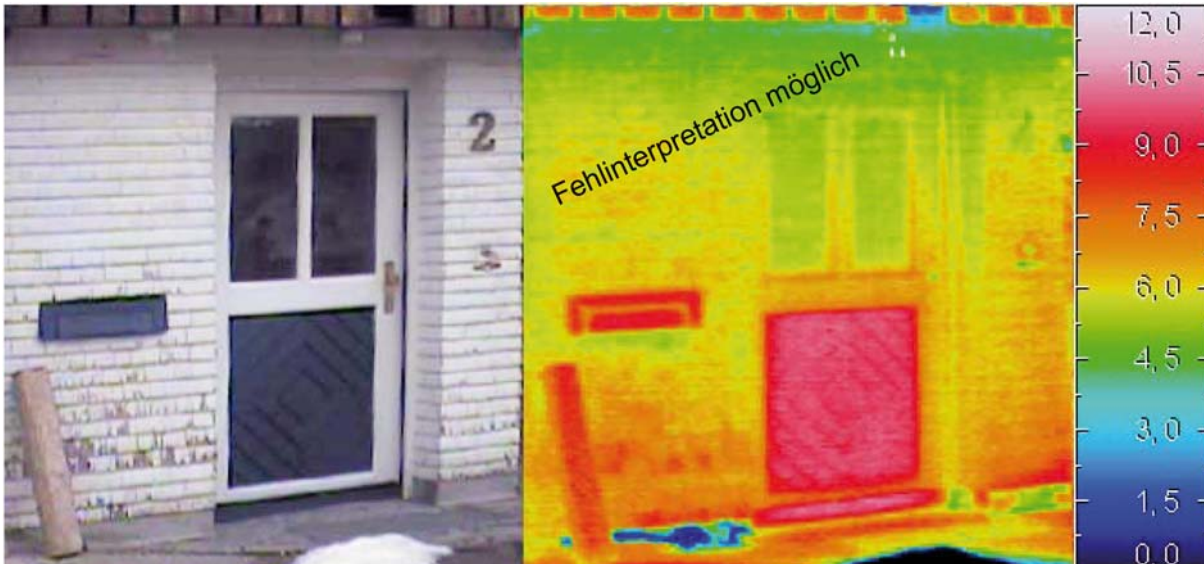
Bild 8 Thermographie einer neuen Außentür in einem Altbau. Die dunklen Flächen werden durch die Absorption des diffusen Tageslichts erwärmt und weisen daher eine höhere Temperatur auf.
