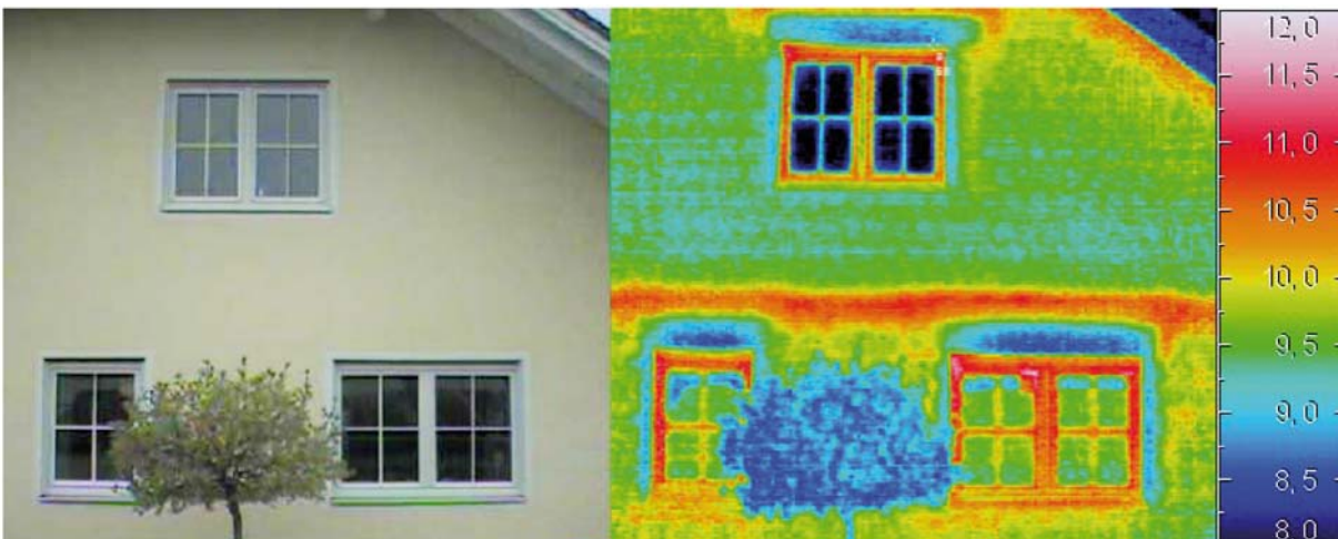
Bild 12 Wärmebrücke Deckeneinbindung
