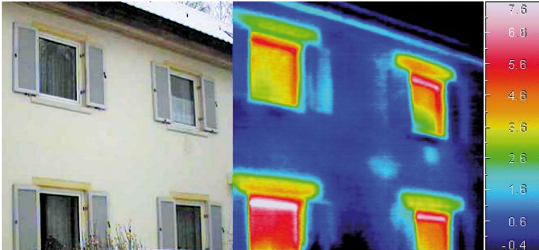
Bild 11 Wärmebrücke Fenstersturz
