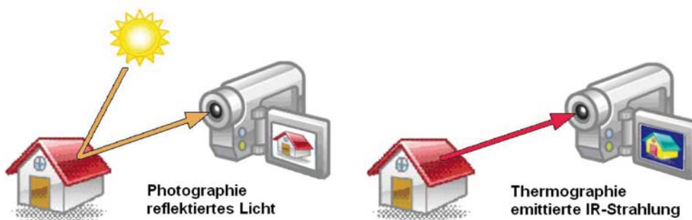
Bild 2 Vergleich von Photographie und Thermographie Die Photographie registriert das vom Objekt reflektierte Licht. Die Thermographie registriert die vom Objekt ausgehende emittierte Infrarot-Strahlung.
