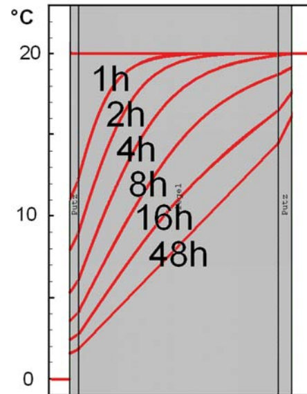
Bild 7 Bei einer plötzlichen Änderung der Außentemperatur wird bei einer massiven Außenwand erst nach 48 h (2 Tagen) ein stationärer Temperaturverlauf erreicht. Bei realen Umweltbedingungen hängt die Oberflächentemperatur von der Geschichte, d. h. von den Bedingungen der letzten Stunden bzw. Tage, ab.
