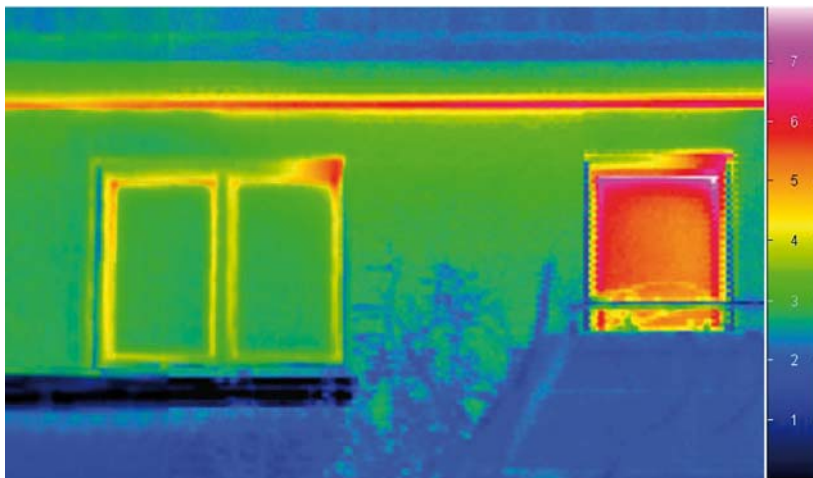
Bild 10 Fenster mit Dreifachglas ( U=0,7 ) und Balkontür mit Zweifachglas ( U=3,0 ) in Außenwand ( U=0,4 ). Oberhalb der Fenster die Wärmebrücke „durchgehende Balkonplatte aus Stahlbeton“. Wegen der identischen Randbedingungen ist ein Unterschied der Verglasung deutlich erkennbar. Ein quantitativer Rückschluss auf die U-Werte ist nicht möglich.
