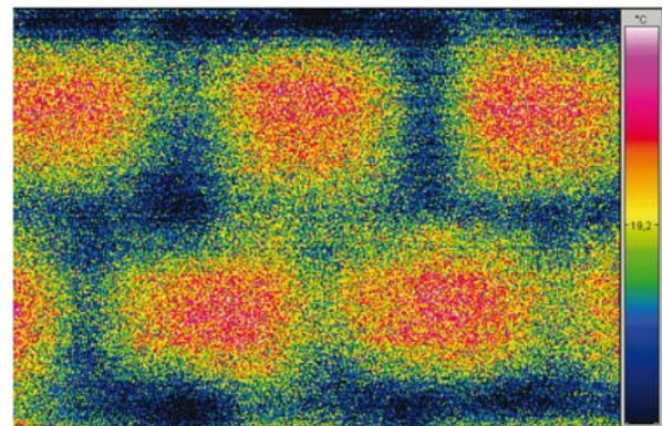
Bild 19 Innere Oberflächentemperatur einer 24 cm Ziegelwand mit 6 cm Außendämmung, Temperaturbereich 19,1 bis 19,3 °C
