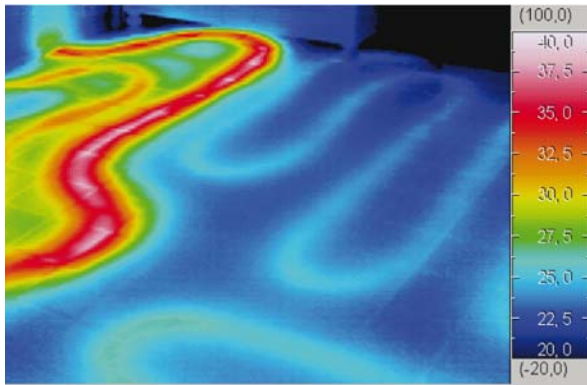
Bild 18 mangelhaft durchströmte Fußbodenheizung
