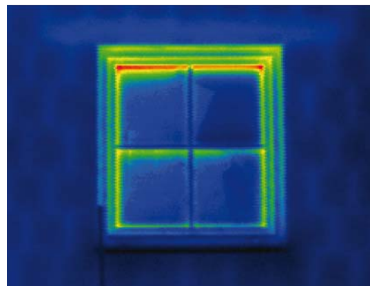
Außenthermographie von „guten“ Fenstern mit Zweifach-Isolierglas.
