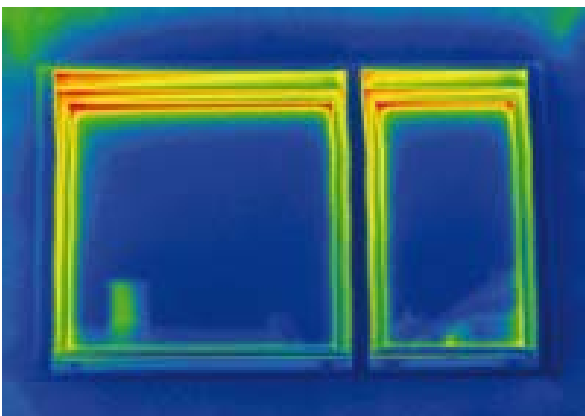
Außenthermographie von „guten“ Fenstern mit Zweifach-Isolierglas.
