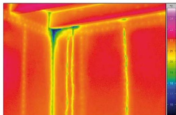
Bild 17 Mit dem Auge nicht sichtbare Feuchtespuren an einer Wand. Durch Verdunstung kühlen die feuchten Bereiche ab und zeigen so das ablaufende Wasser an. Im vorliegenden Fall war das Flachdach undicht.
