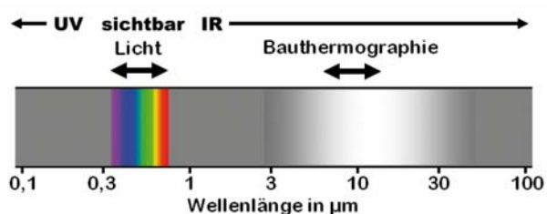
Bild 3 elektromagnetische Strahlungen Der in der Bauthermographie genutzte Bereich liegt im mittleren Infrarot bei 8 bei 12 µm.
