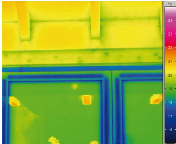
Bild 13 Dreikammer-Kunststofffenster, die Stahlaussteifungen in der raumseitigen Kammer sind deutlich sichtbar und führen zu niedrigeren Temperaturen an der Oberfläche, diverse Reflexionen im Glas werden von Raumleuchten verursacht.
