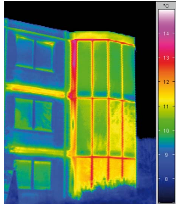
Bild 1 Thermogramm – Außenansicht eines Bürogebäudes mit Glasfassade
