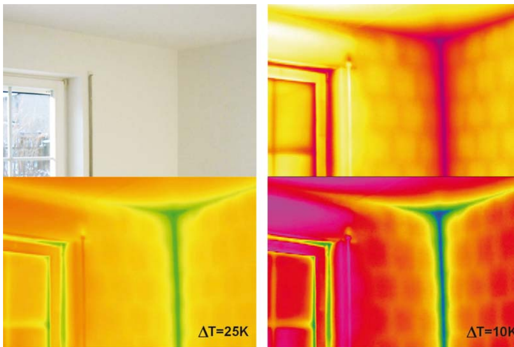
Bild 6 Innen-Thermographie oben links: Gebäudeaußenkante vom Innenraum gesehen, Thermogramme in unterschiedliche Falschfarbendarstellung bei jeweils gleichem Temperaturniveau oben rechts: „Eisenglühfarben“ mit Temperaturbereich 10 K unten: „Regenbogen“ mit Temperaturbereich von 25 K bzw. 10 K
