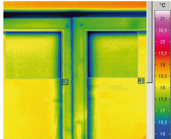
Bild 14 Unterschied in der Oberflächentemperatur zwischen thermisch verbessertem Randverbund und Standard-Randverbund von Zweischeiben-Isolierglas U=1,1 (Emissionsgrad-Korrektur in den Feldern R1 und R2)
