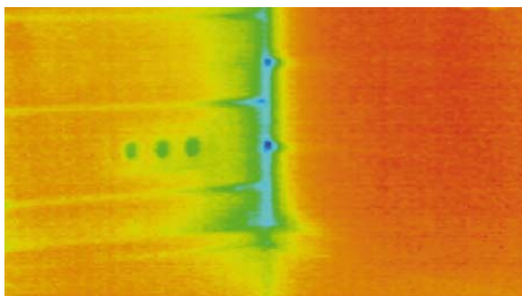
Bild 15 Leckagen bei einem Holzgebäude in Blockbauweise. links: Thermographie bei Normalbedingung Die Ursache der Leckage, Fehlstellen in der Luftdichtheitsschicht, ist damit noch nicht gefunden.
