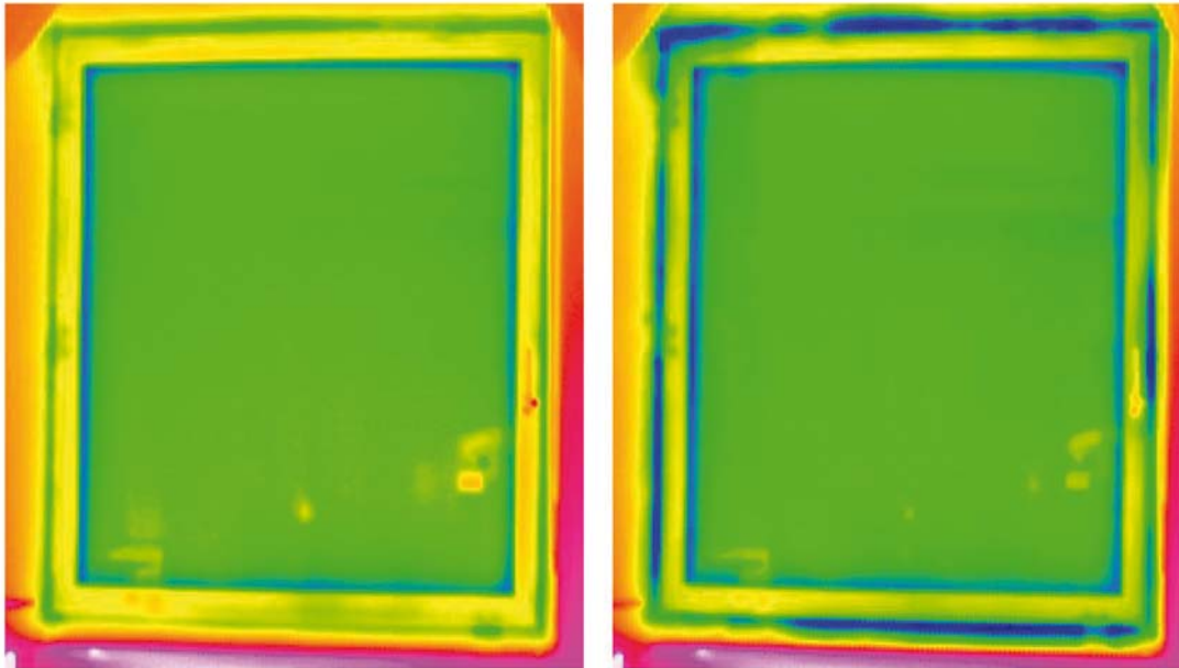
Bild 16 Die Kombination von Blower-Door und Differenz-Thermographie ist zum Nachweis und zur Ortung von Leckagen bestens geeignet. links: Fenster bei niedriger Außentemperatur und Normalbedingungen. rechts: gleiches Fenster bei Unterdruck nach 10 Minuten. Die einströmende Kaltluft kühlt die Oberflächen und wird durch Vergleich mit der vorherigen Aufnahme sichtbar. Eine quantitative Aussage über die Luftdichtheit des Fensters ( \alpha -Wert) ist damit nicht möglich. Sofern andere Leckagen ausgeschlossen werden, kann dies nur durch Auswertung der Blower-Door-Messung geschehen.
